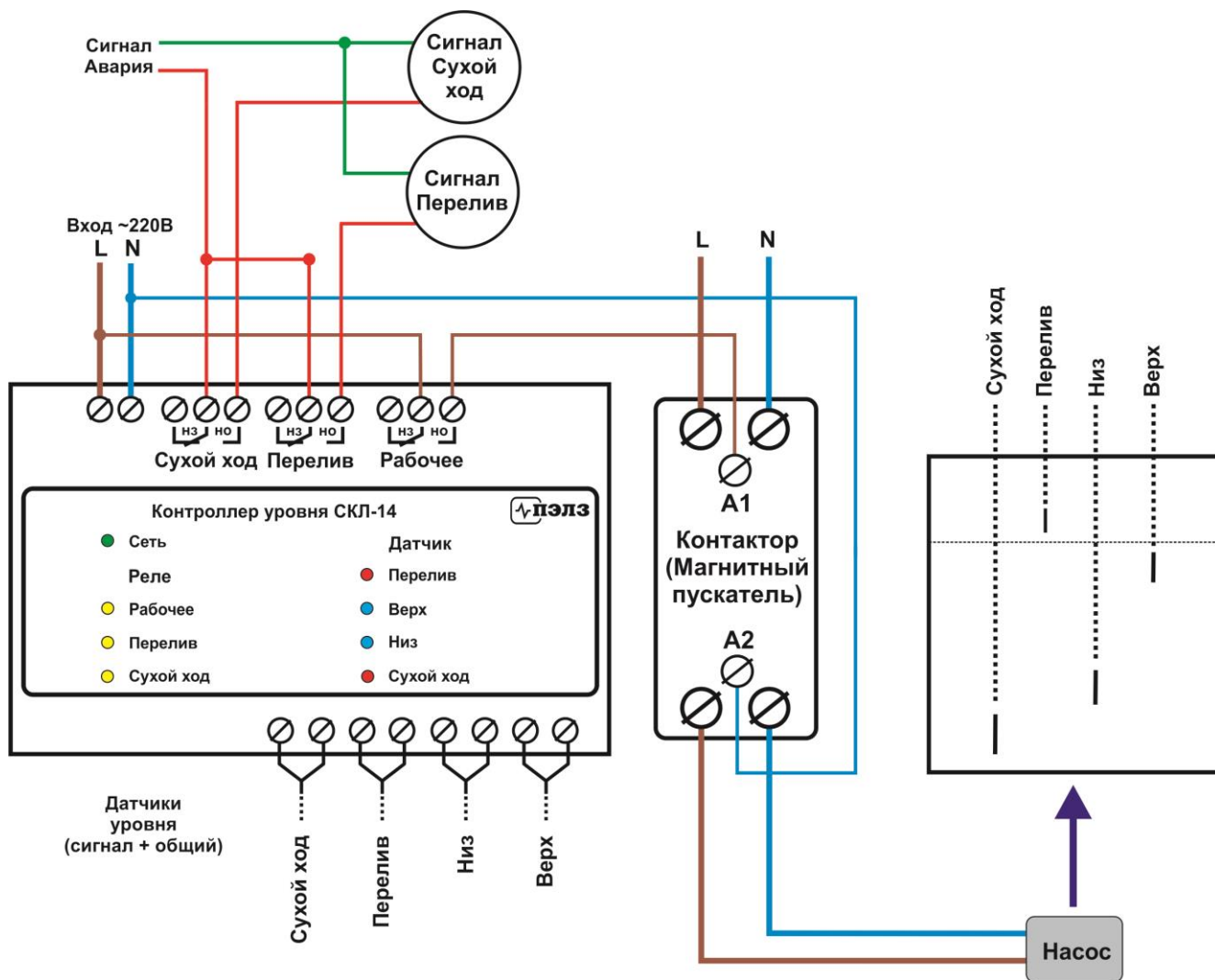
Рис. 1. Вариант схемы подключения контроллера СКЛ-14 для организации системы пополнения расходного бака.
