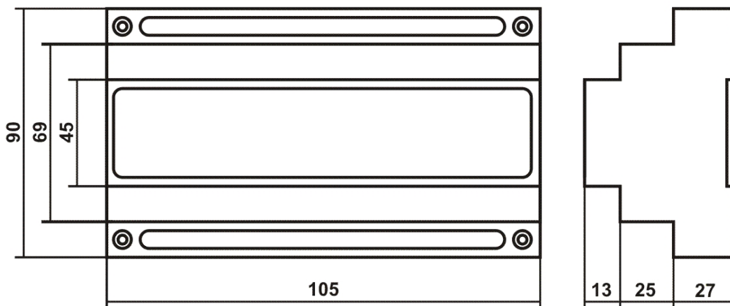
Рис.2. Габаритные размеры прибора.
