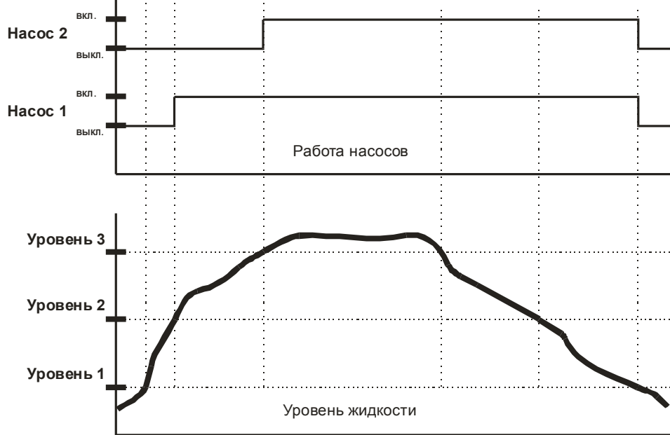
Рис.2. Диаграмма работы контроллера уровня.
